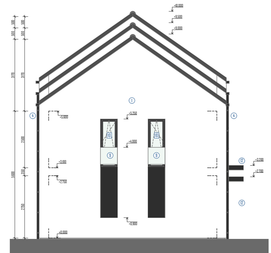
SO-107_POHLED SEVERNÍ
