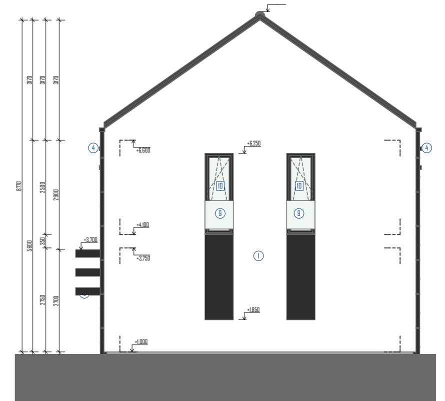
SO-107_POHLED JIŽNÍ
